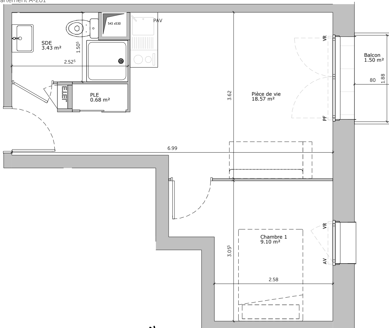
Plan de repérage appartement A-201
