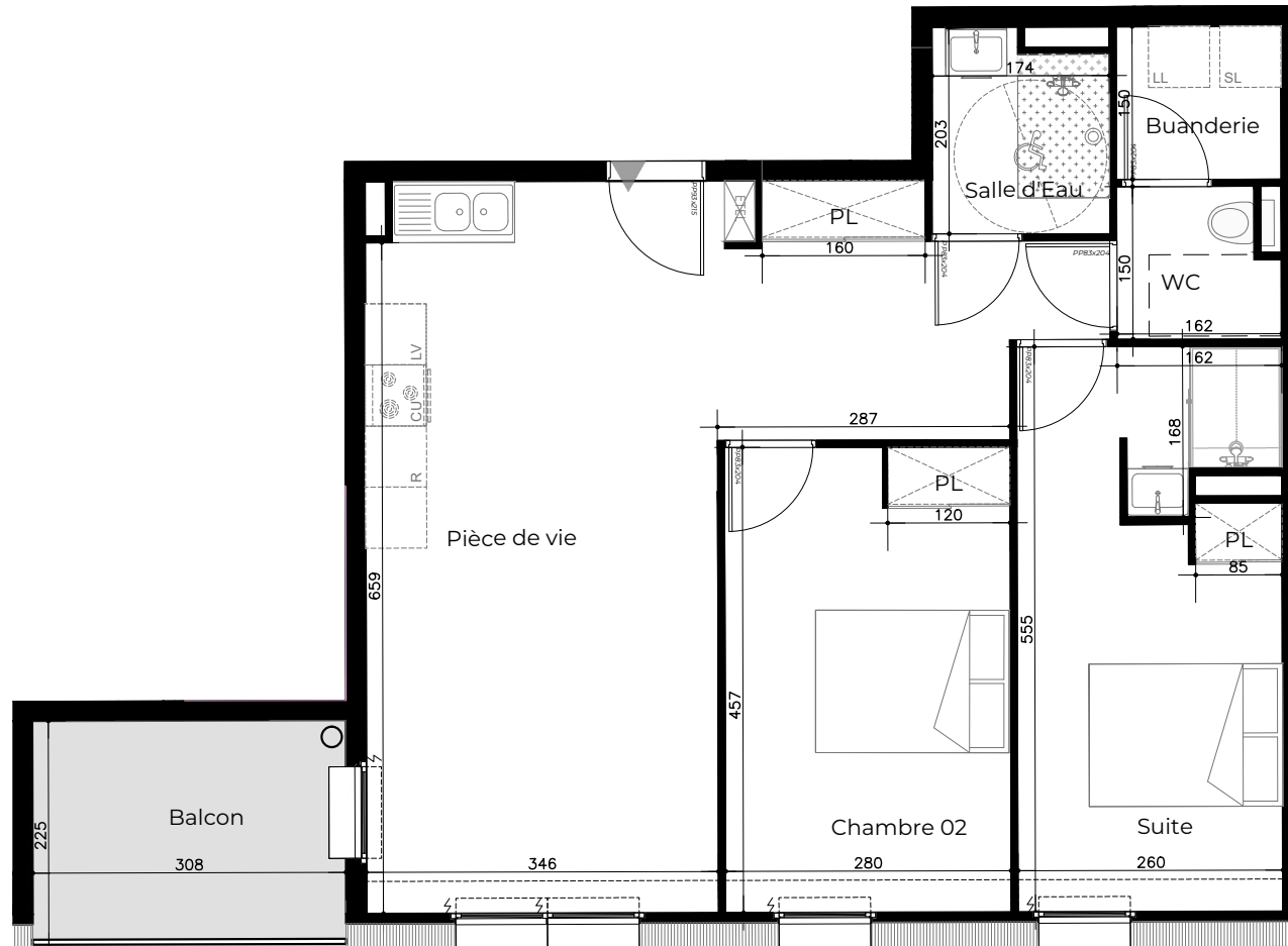
Plan de repérage / R+3 - Attique Appartement A301
