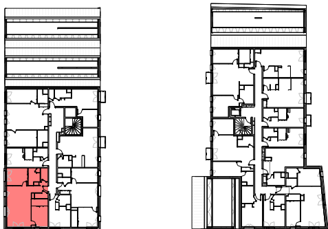
Plan de repérage appartement A-304
