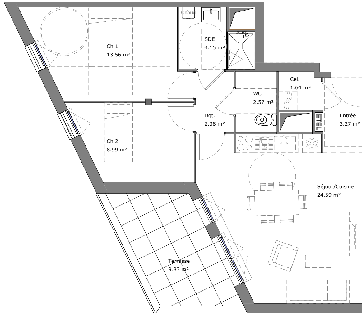
Plan de repérage appartement B_103
