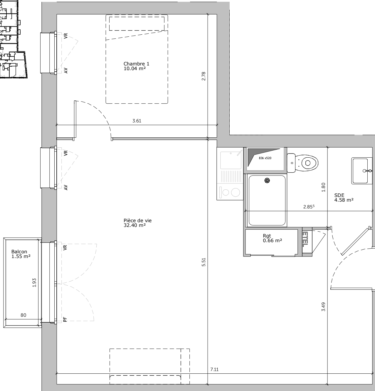
Plan de repérage appartement B-201
